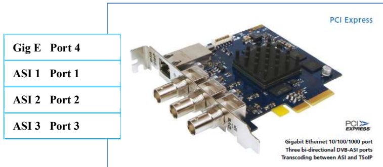
Figure: DekTec card
