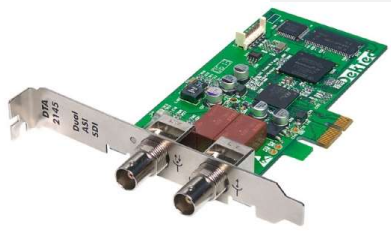
Figure: DekTec DTA-2145
